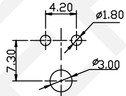
02P P.C.B Layout
